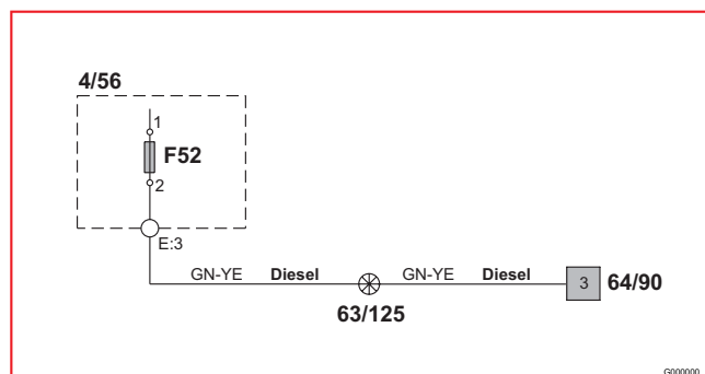
63/125 MPS6 柴油引擎
